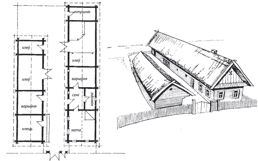
• Прыклад двухраднага пагона, агульны выгляд і план (в. Валеўка Навагрудскага раёна)
