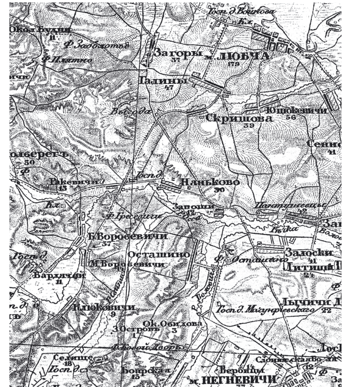
• Асташына і наваколлі на тапаграфічнай карце 1865–1866 гг. Крыніца: http://www.etomesto.ru/shubert-map/15-5/
